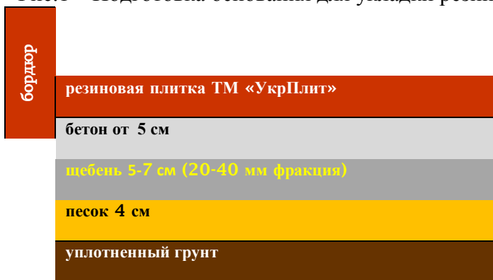
Рис.1 – Подготовка основания для укладки резиновой плитки на бетон:
